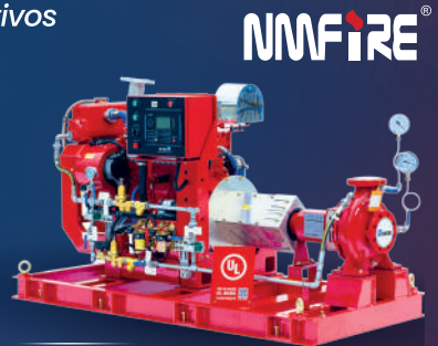
Sistemas Contraincendio
